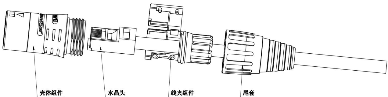
装配示意图
