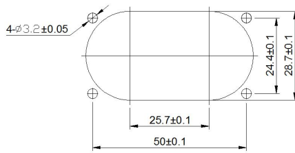
面板开孔尺寸
